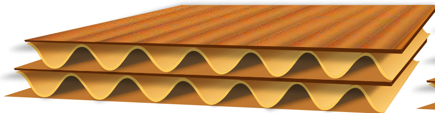
5-слойный картон (3 лайнера и 2 флютинга)
