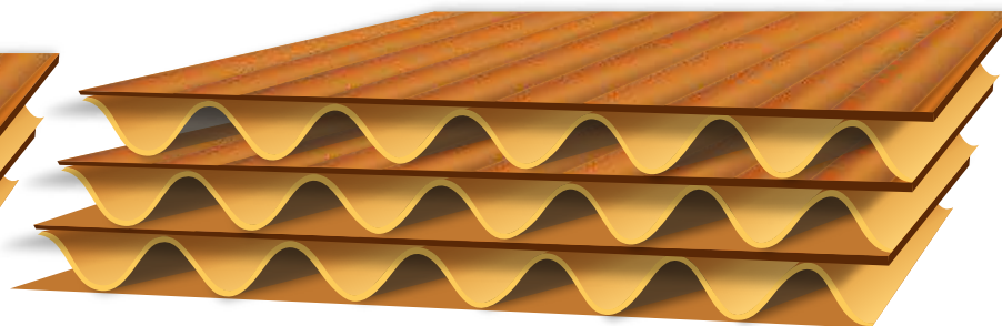
7-слойный картон (4 лайнера и 3 флютинга)
